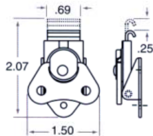
622-60 Long base
