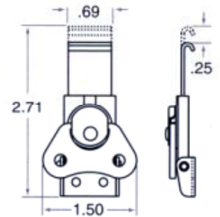
622-29 Long hook
